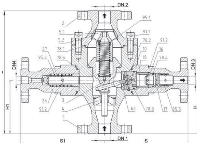
Abbildung 3: SMV 18 Schnittbild
